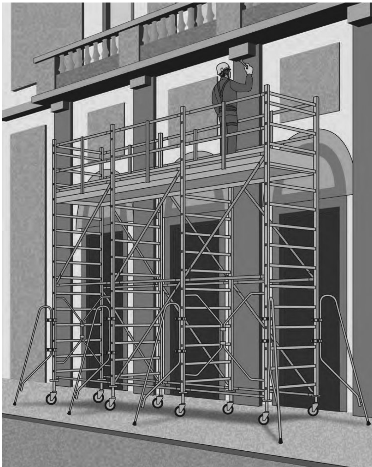
Figura 5 - Utilizzo di un trabattello multiplo (se previsto dal fabbricante)
