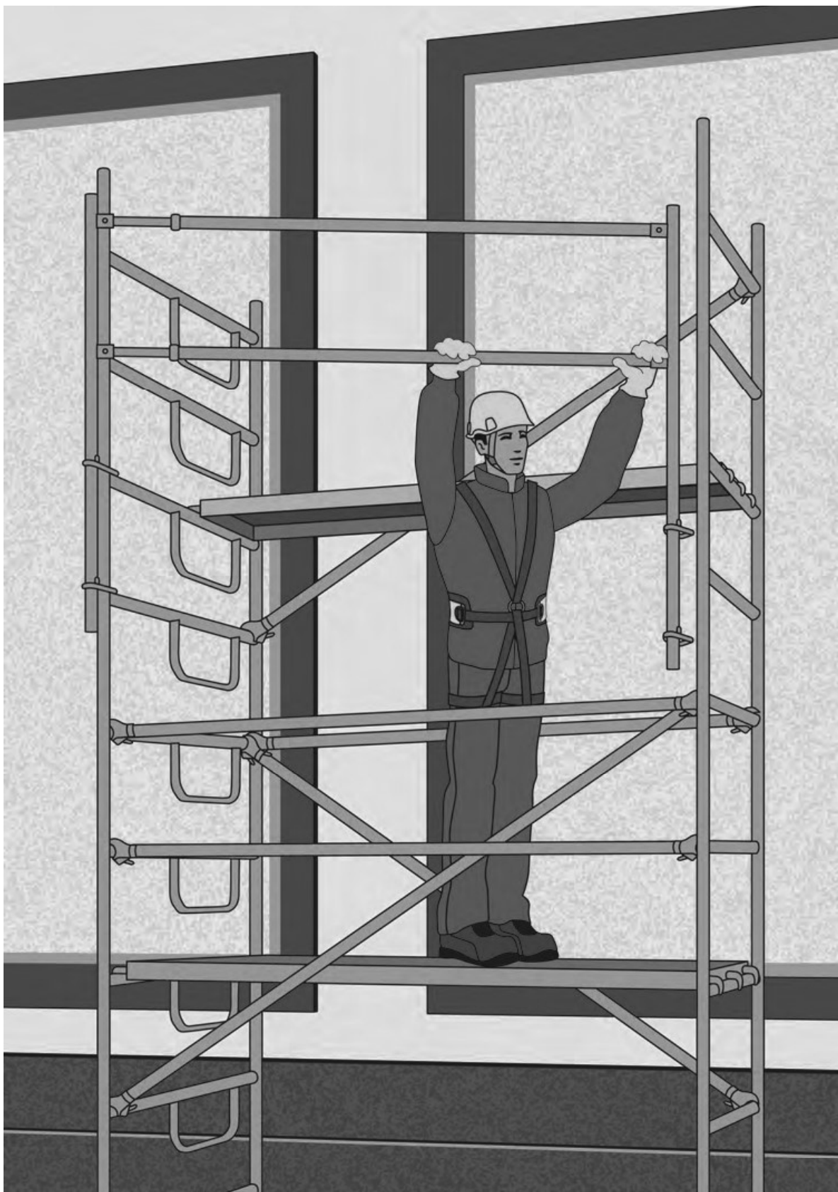
Figura 4 - Trabattello con montaggio dal basso
